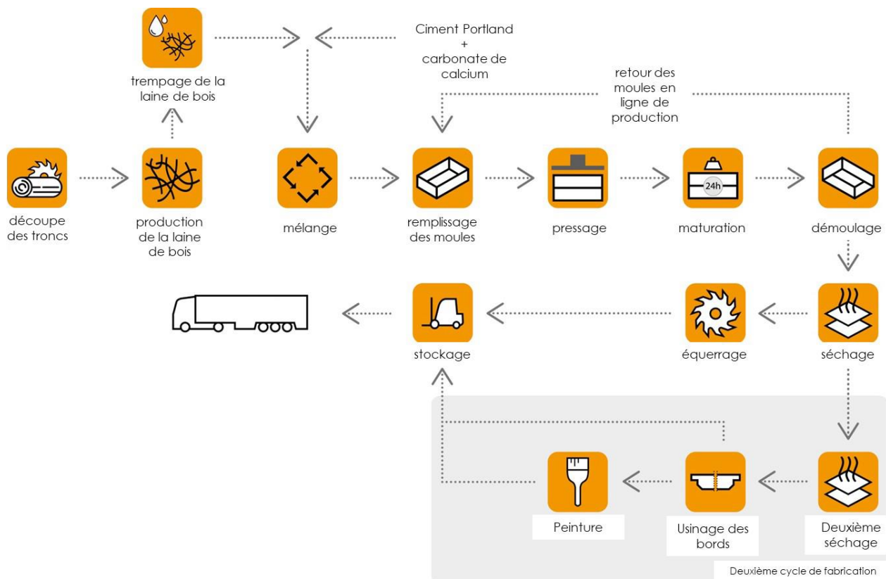
Figure 1 : Schéma du procédé de fabrication des panneaux PUREBEL, avant assemblage avec la laine de roche
