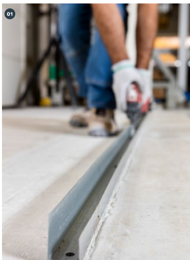
POSE DU RAIL SECURBLOCK R30 EN PARTIE BASSE
