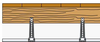
Avec Fourrure et entretoise S47
